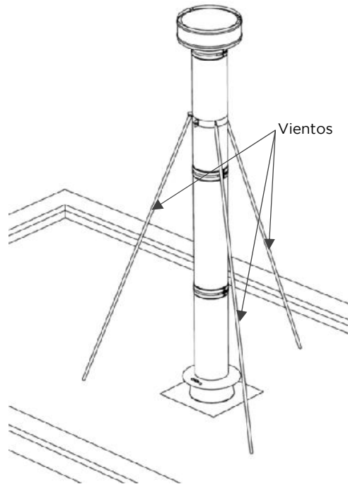
Figura 2.12, Abrazadera de vientos (542)
