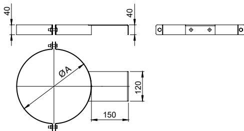
ABRAZADERA CON PLETINA
